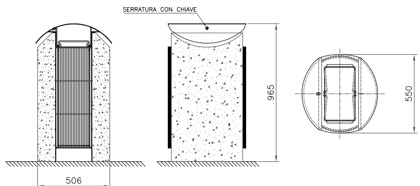
Versione in tondino con coperchio
